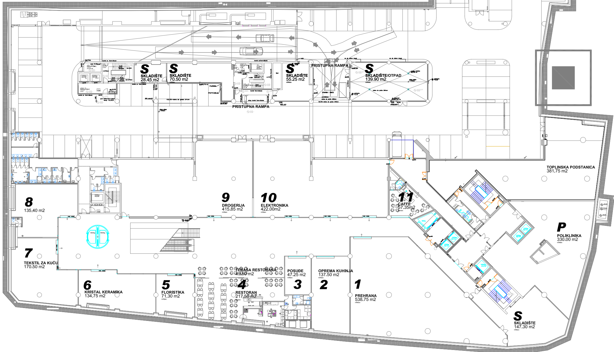
EURODOM OSIJEK TLOCRT PODRUMA
